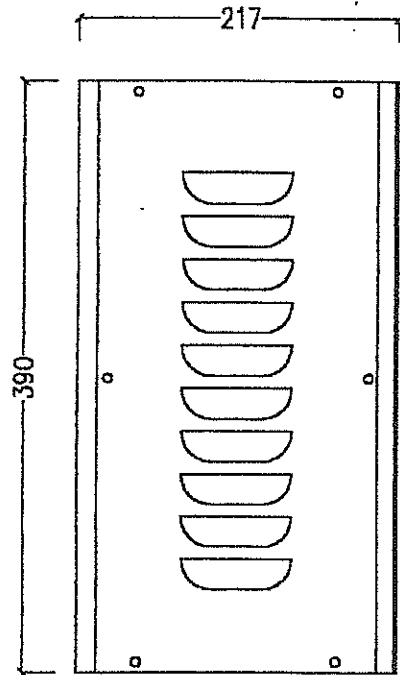
SCALE 1 : 5
