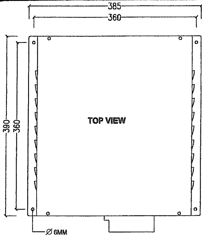
SCALE 1 : 5
